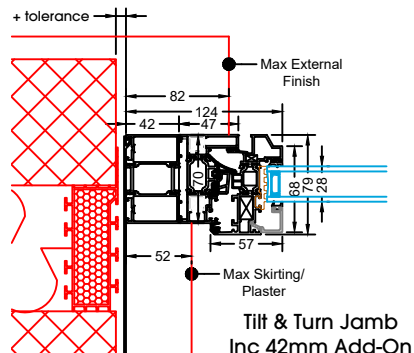
Tilt & Turn Jamb
