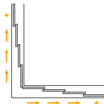
Abwinklung 90° Corner angles 90°
