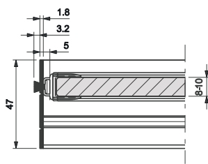
Mit Bürstendichtung With brush gasket
